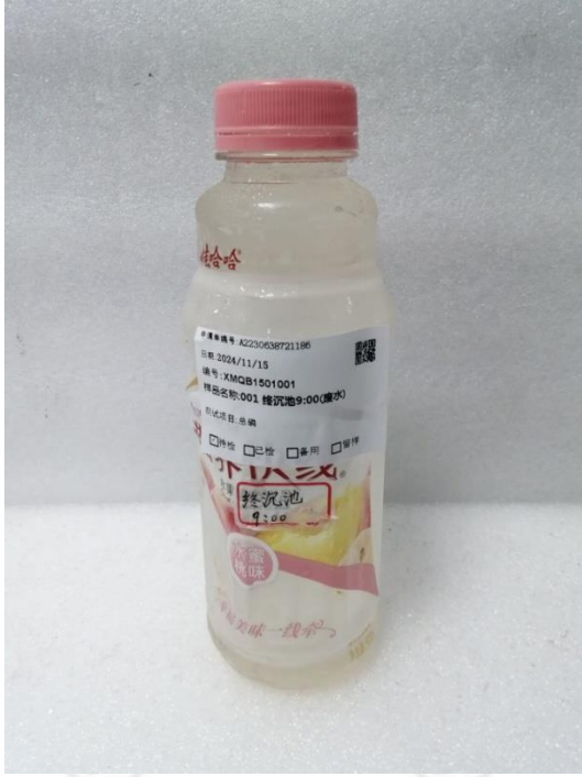
终沉池 9:00
